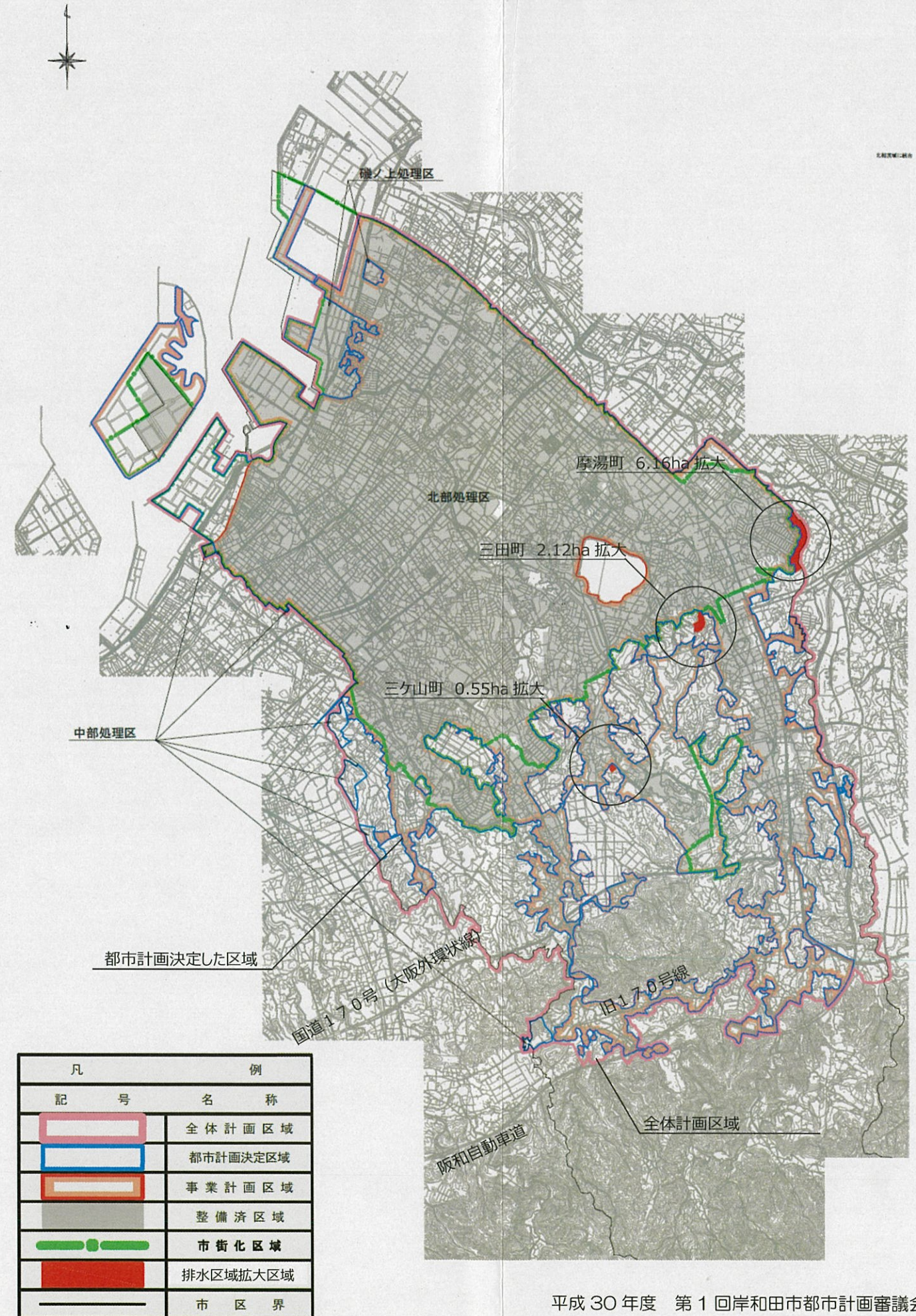
汚水整備状況図及び排水区域の拡大箇所図
