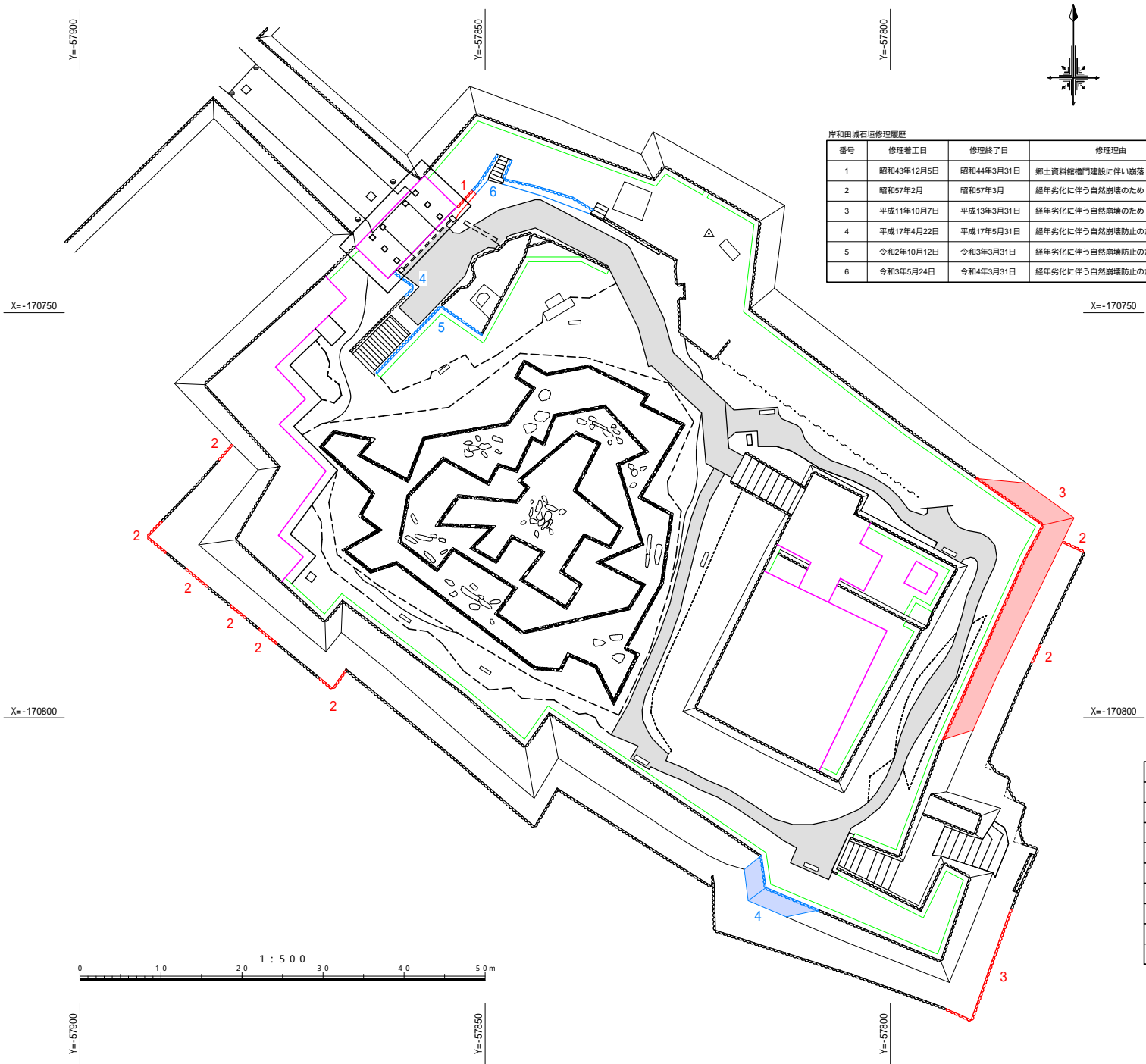
[ 図2 ] 岸和田城石垣修理位置図
